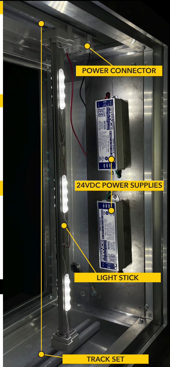
24VDC QUATTRO TRULUME LEDs
